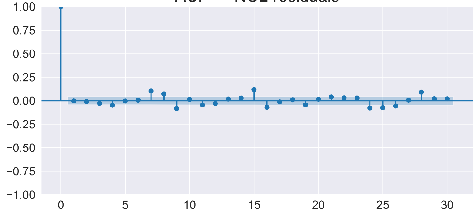
ACF — NO2 residuals
